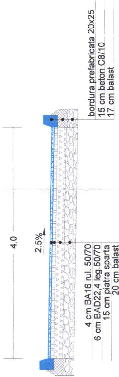
Detaliu alee carosabila Scara 1:10
