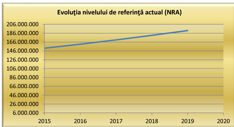
Fig. 1.6 Evoluția NRA
